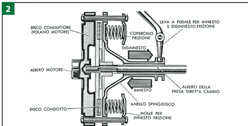
Fig. 2. Schema di innesto a frizione monodisco (Fiat).
