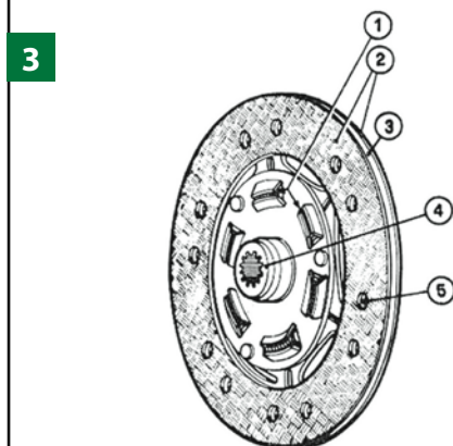
Fig. 2. Schema di innesto a frizione monodisco (Fiat).
