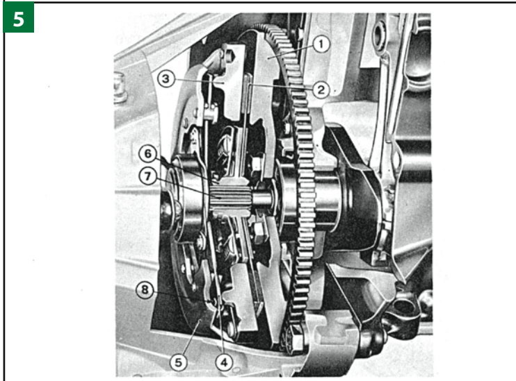
Fig. 6. Frizione monodisco a secco con comando meccanico (Renault): 1) Volano motore; 2) Disco condotto; 3) Anello spingidisco; 4) Molla a diaframma; 5) Coperchio frizione; A) Cuscinetto reggispinta; B) Leva a forcella; C) Cavo collegato al pedale comando frizione. Quando si preme sul pedale della frizione la leva a forcella B spinge il cuscinetto reggispinta A contro la molla 4, provocando così l'inversione della concavità di quest'ultima, e quindi il disinnesto della frizione.
