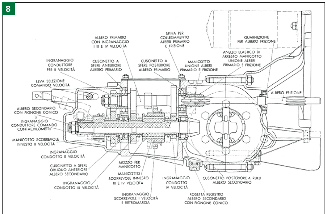
Fig. 8. Sezione longitudinale del complessivo cambio di velocità-differenziale.
