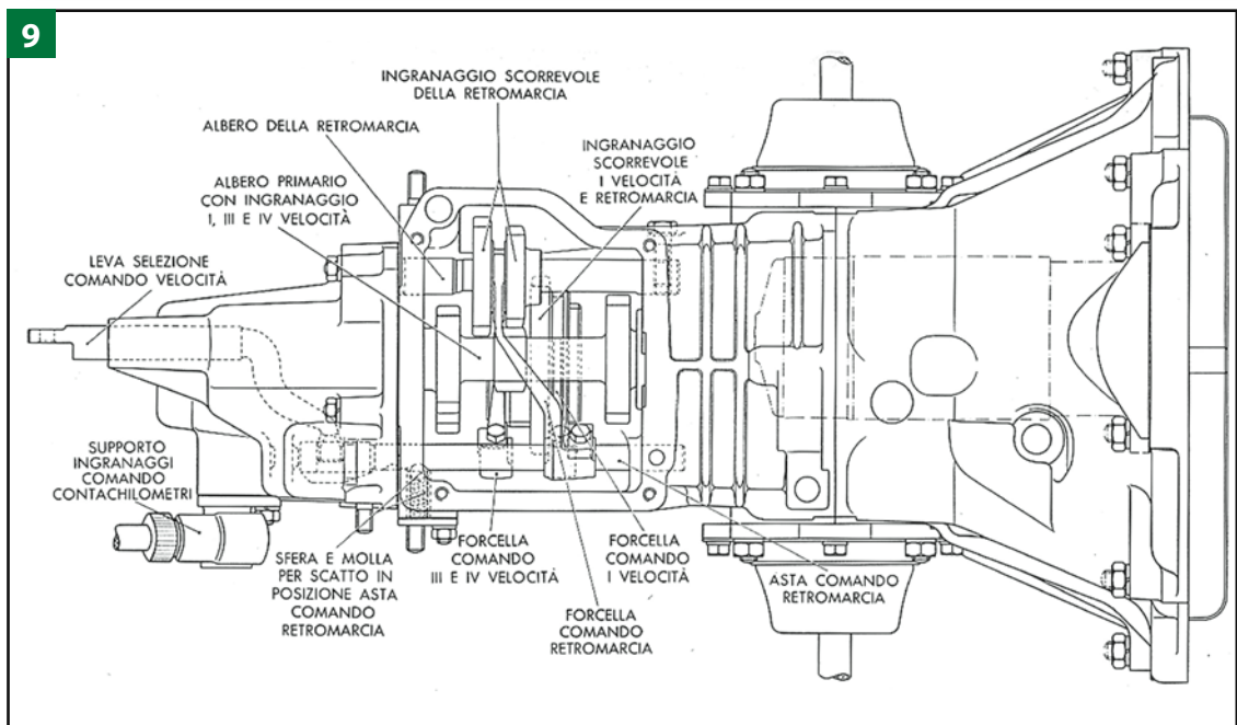
Fig. 9. Complessivo cambio di velocità-differenziale, visto dall'alto, senza il coperchio d'ispezione degli ingranaggi.
