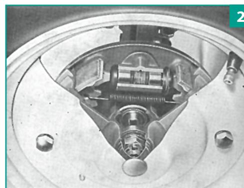
Fig. 2. Sezione parziale sul cilindro e sul mozzo di una ruota anteriore.
