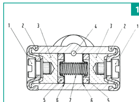
Fig. 1. Sezione di un cilindro comando ganasce.
