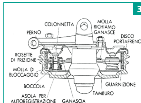
Fig. 3. Sezione complessiva freni della ruota anteriore sinistra, sul dispositivo autoregistrante.
