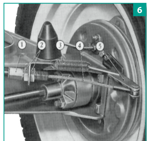
Fig. 6. Comando del freno a mano di sicurezza applicato ad una ruota posteriore.
